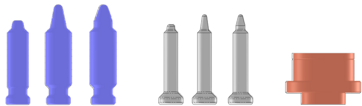
Illustration exemplaire de gauche à droite : épingles de centrage Cerazur M12 courtes, longues et avec col ; Les goupilles de centrage Volcera M4 sont courtes, longues et avec col ainsi qu'une entrejambe en cuivre interchangeable.
