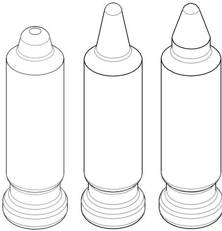
Illustration fidèle à l'échelle des variantes à épingle de centrage de la taille M8 courte, longue et avec col.
